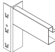
SSS Step Beam 45X80
